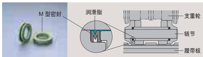
M 型履带链节密封使润滑脂的密封性能大幅度提高
