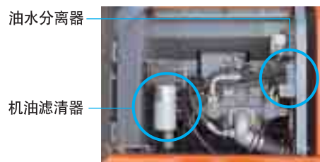
机油滤清器和油水分离器的安装位置便于站在地上进行检查
