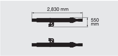
动臂油缸 550 kg×2 总高度：410 mm
